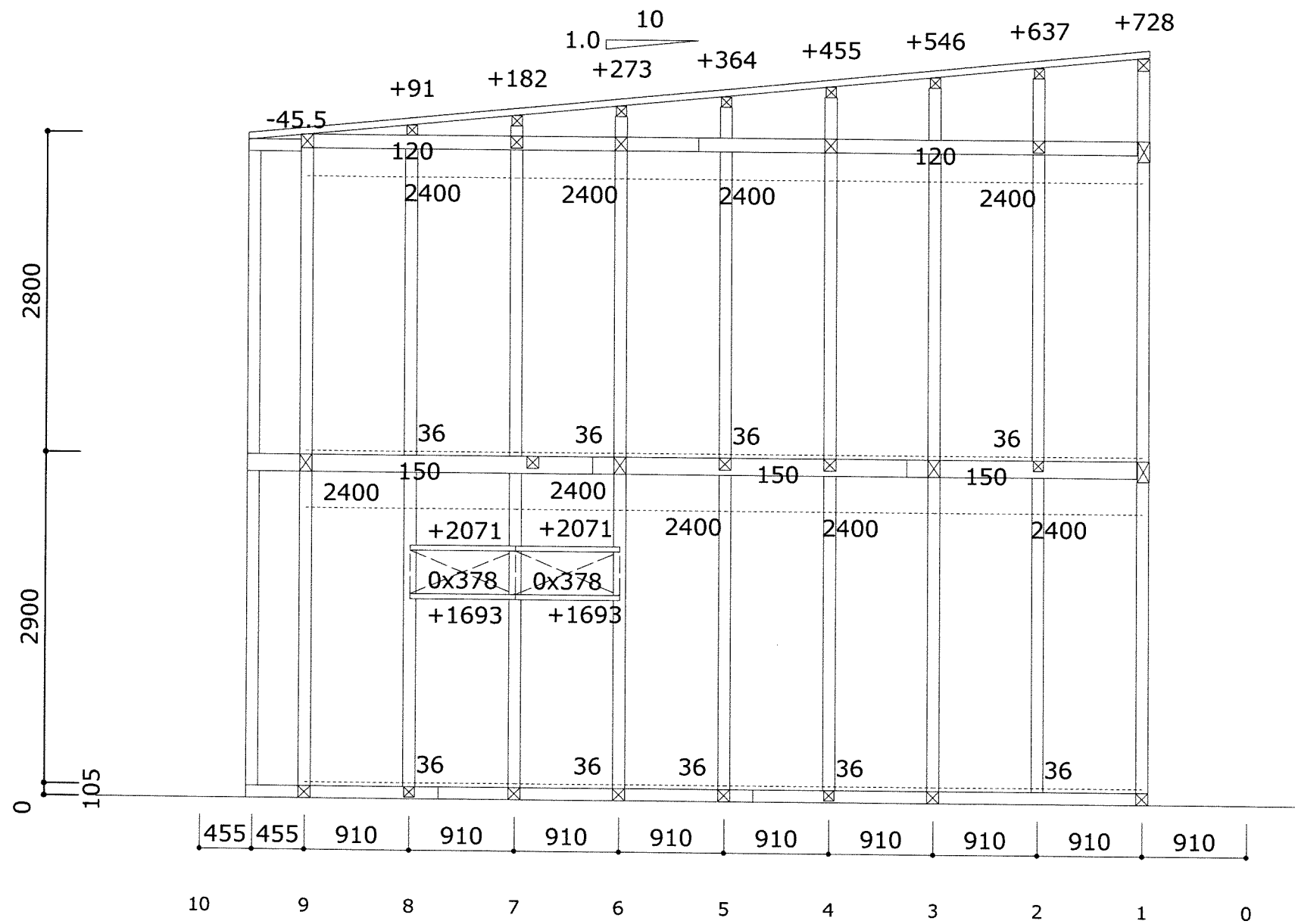
り通り 東面
