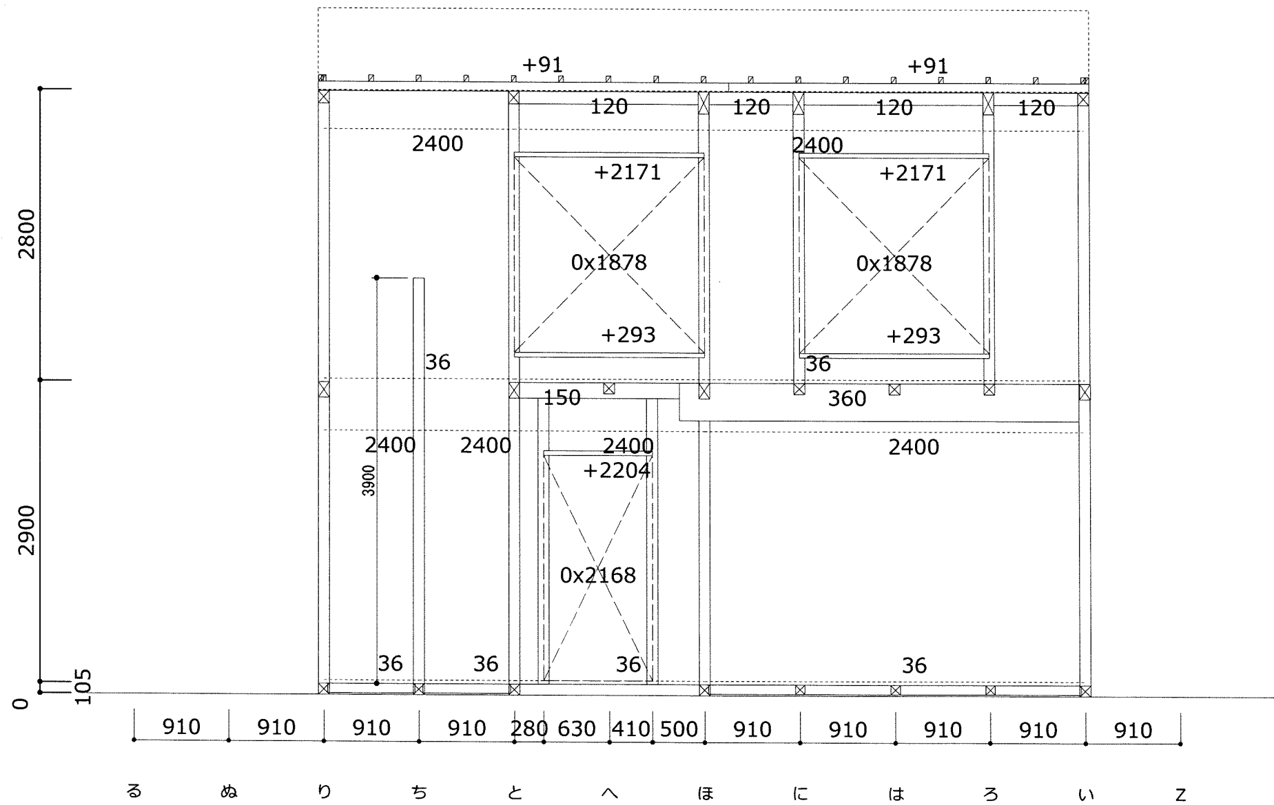
8通り 南面
