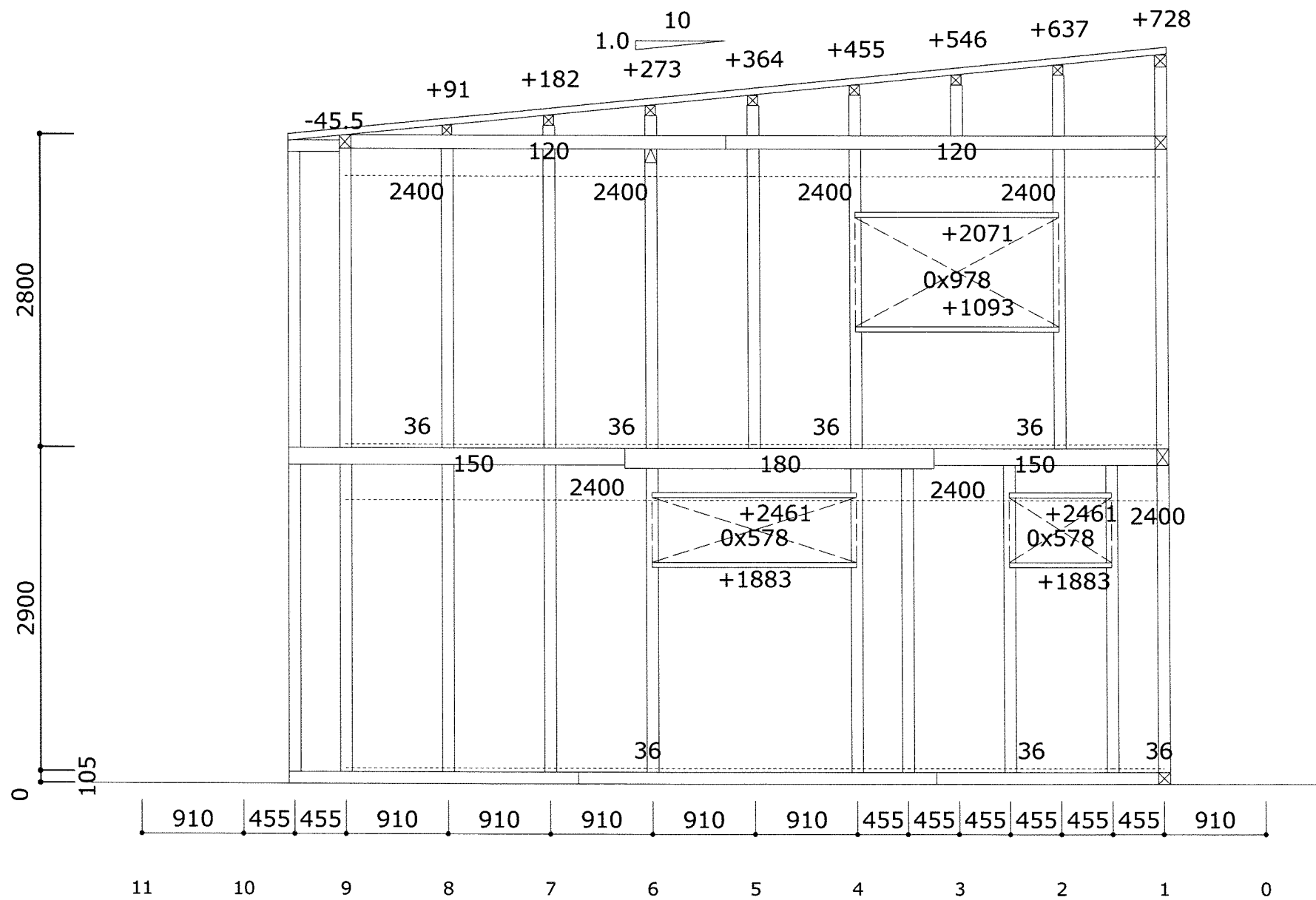
い通り 東面
