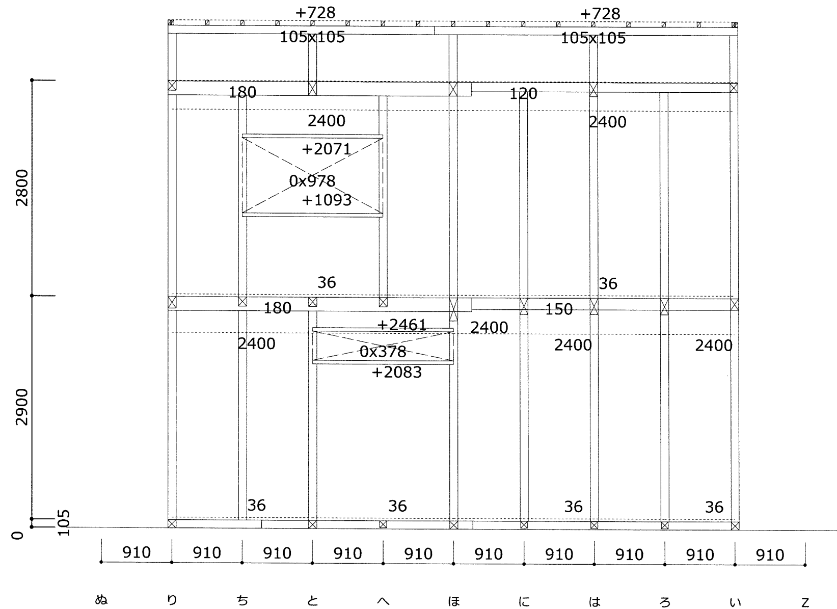
1通り 南面
