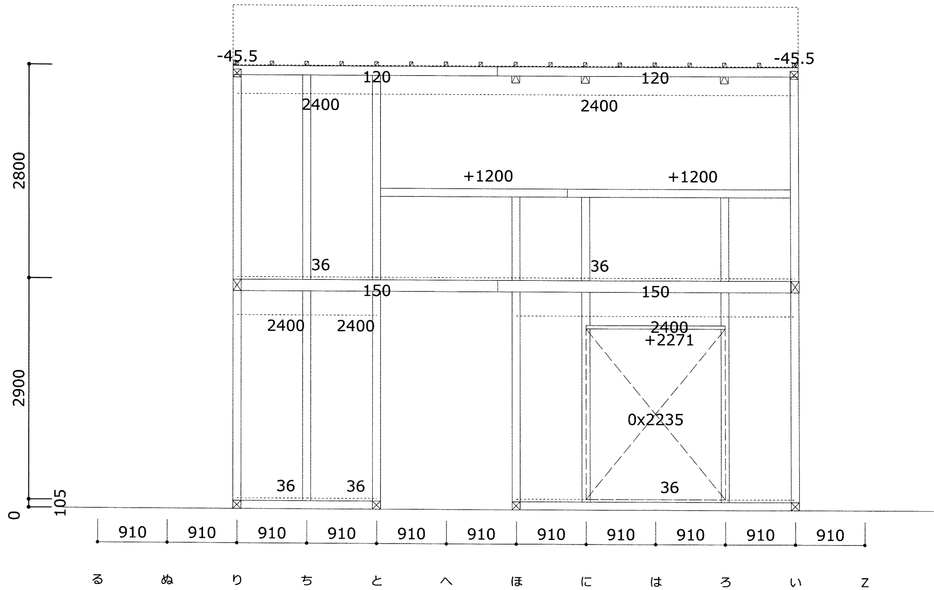
9通り 南面
